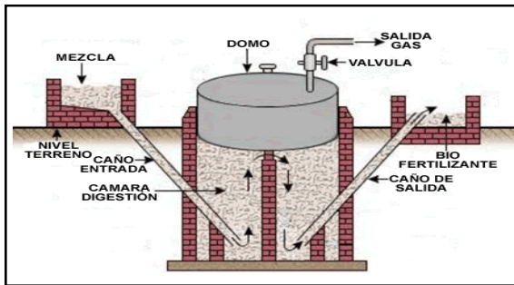
FIG 3: Biodigestores tipo hindú
