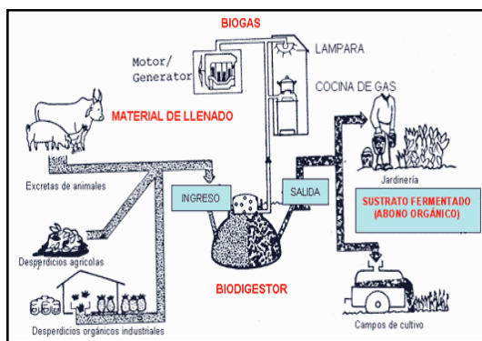
Figura 1. Ciclo de la biomasa en los biodigestores
