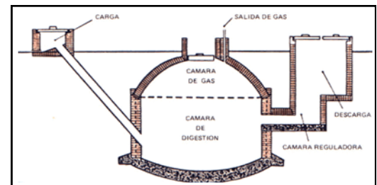
FIG 2: Biodigestores tipo chino
