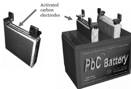
Figura 1.3 Batería PbC [14].
