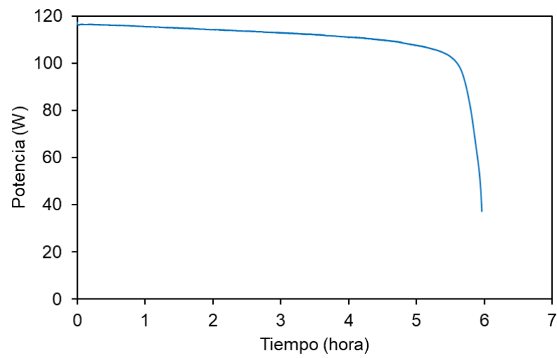
Figura 3.2 Curva de potencia-Batería Champion 27MDC (nueva).
