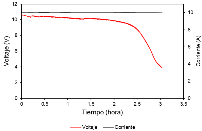
Figura 3.5 Curva de descarga de una batería cale 31T
