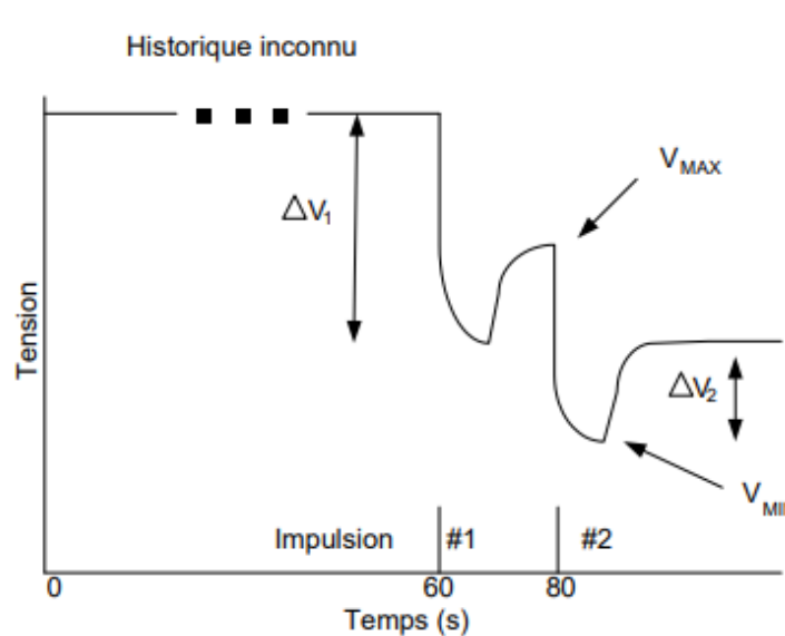
Figura 1.4 Variación de voltajes en el método de dos pulsos [19].
