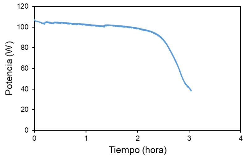
Figura 3.6 Curva de potencia de una batería Cale 31T
