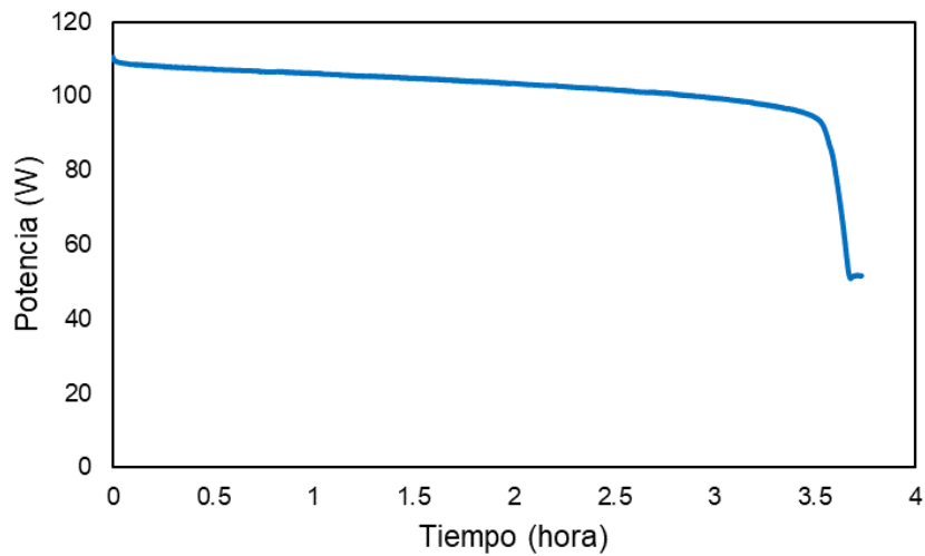
Figura 3.8 Curva de potencia de una batería marca US 182HC XC2.
