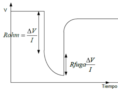
Figura 1.7 Representación de resistencia óhmica y de fuga en la respuesta de una batería a una corriente [20].
