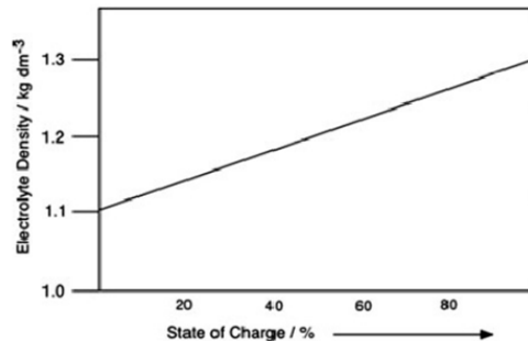
Figura 1.6 Relación entre la densidad del electrolito y el SOC [20].
