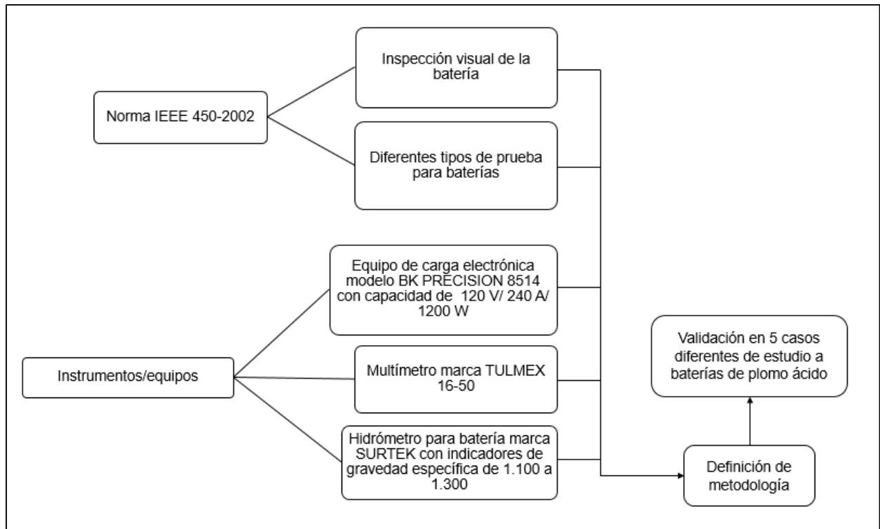
Figura 2.1 Diagrama de flujo para definir la metodología de carga/descarga para baterías plomo ácido.
