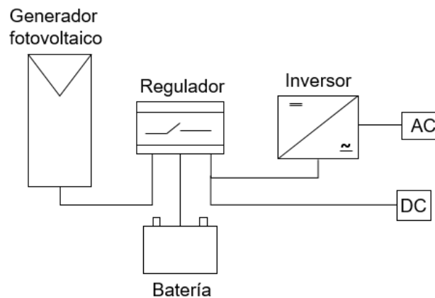
Figura 1.1 Sistema de conexión de un sistema fotovoltaico.
